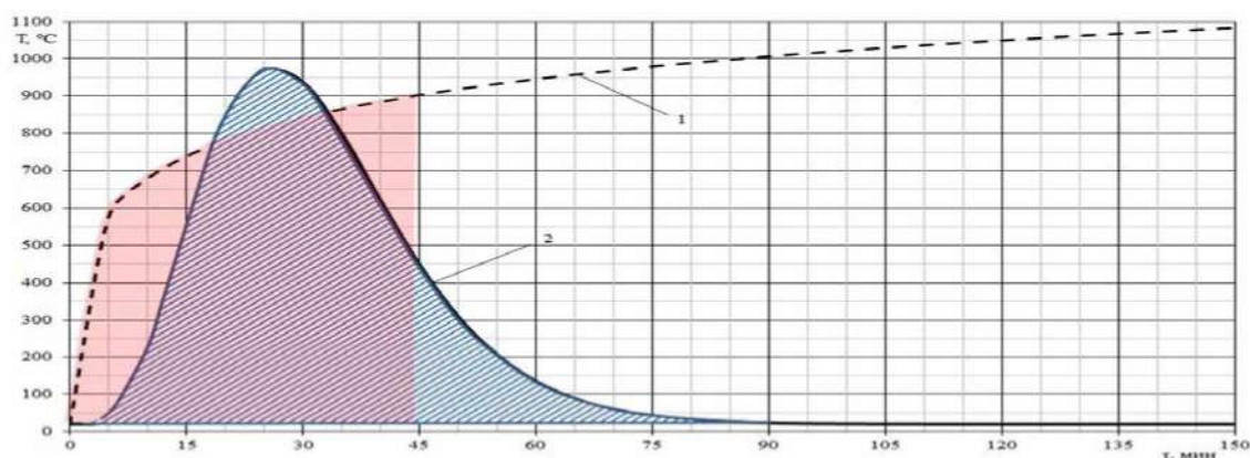
1 – стандартный пожар по ГОСТ 30247 [6]; 2 – среднеобъемная температура по СТБ 11.05.03 [5]
