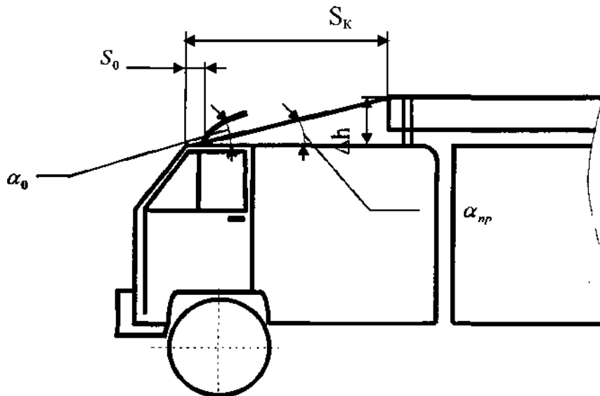
Рисунок 2 – Схема расположения обтекателя
