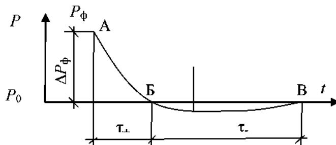
Рисунок 1 – Изменение давления в фиксированной на местности точке при прохождении волны избыточного давления [2].
