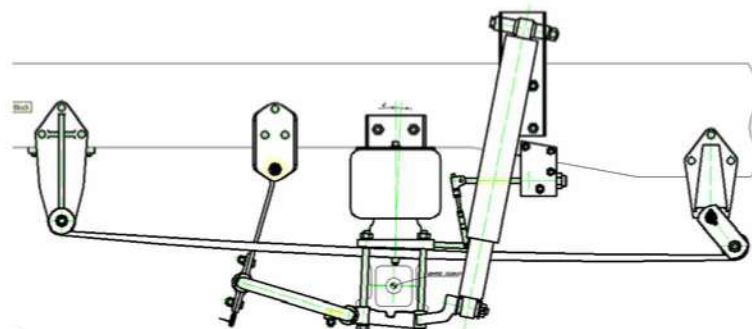
Рисунок 1 – Передняя рессорно-пневматическая подвеска МАЗ-4370
