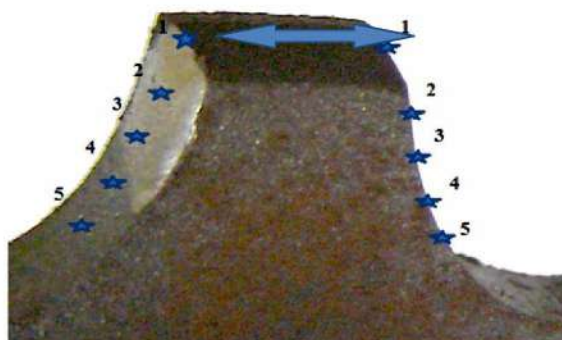
Рисунок 1 – Позиции и направление замеров на зубьях реборды барабана
