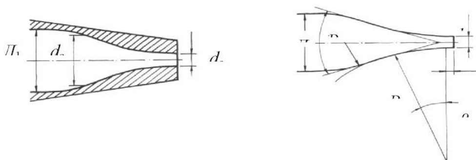
Рисунок 1 – Схема замены гиперболического профиля сопла соответствующим радиусом
