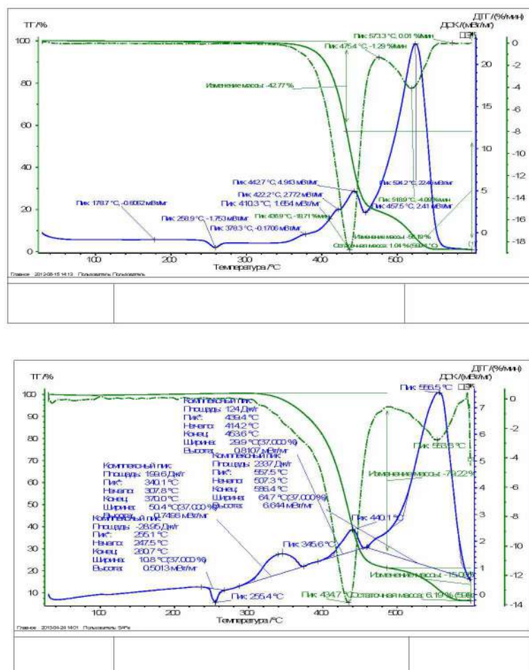
Рисунок 1 – Термогравиметрические кривые в присутствии кислорода для полиэфирного материала до и после ступенчатой огнезащитной обработки
